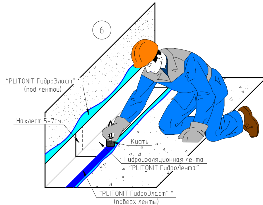
Рис.32.1. Последовательность работ (на стенах работа в аналогичном порядке), где: 1 - проверка ровности основания контрольной рейкой (аналогично для горизонтальной поверхности); 2 – размещение емкости с мастикой; 3 – нанесение первого слоя мастики, разбавленной водой в пропорции 1:10, на основание; 4 – нанесение гидроизоляции на поверхность (аналогично для горизонтальной поверхности); 5 – укладка гидроизоляционной ленты на поверхность, предварительно обработанную «PLITONIT ГидроЭласт» или «PLITONIT WaterProof Standard»; 6 – поверхностная обработка ленты мастикой «PLITONIT ГидроЭласт» или «PLITONIT WaterProof Standard»
