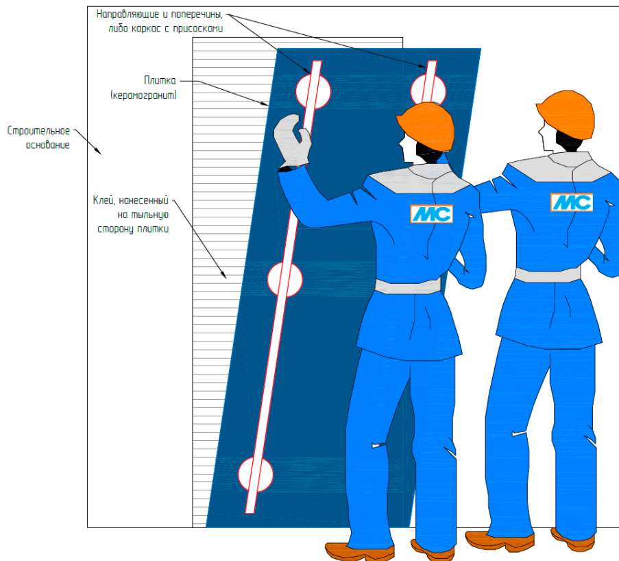
Рис. 38. Монтаж крупноформатного керамогранита
