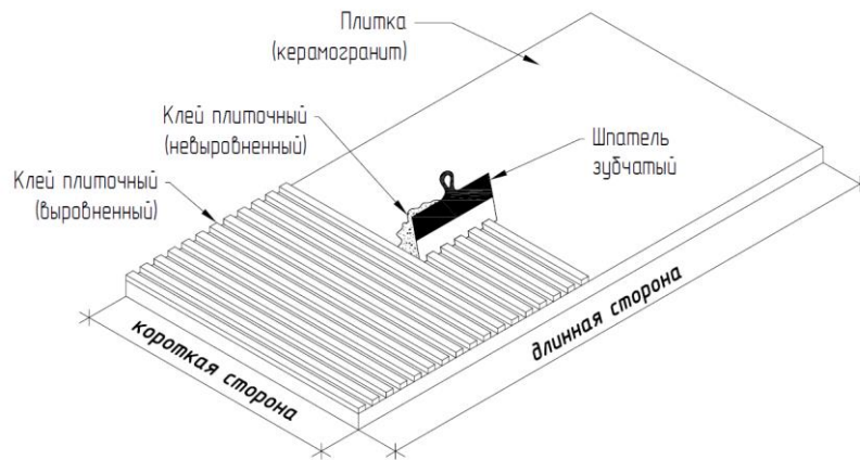
Рис. 33. Нанесение плиточного клея на плитку
