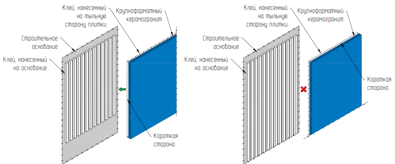
Рис. 34. Клей следует наносить в одном направлении на основание и на плитку
