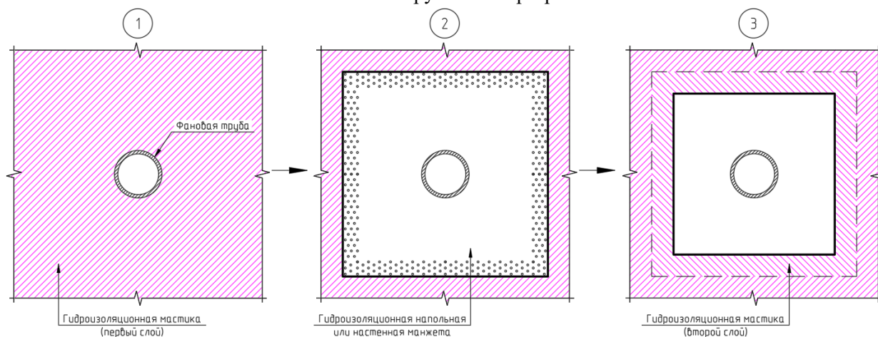
Рис.31.4. Последовательность нанесения гидроизоляционной манжеты
