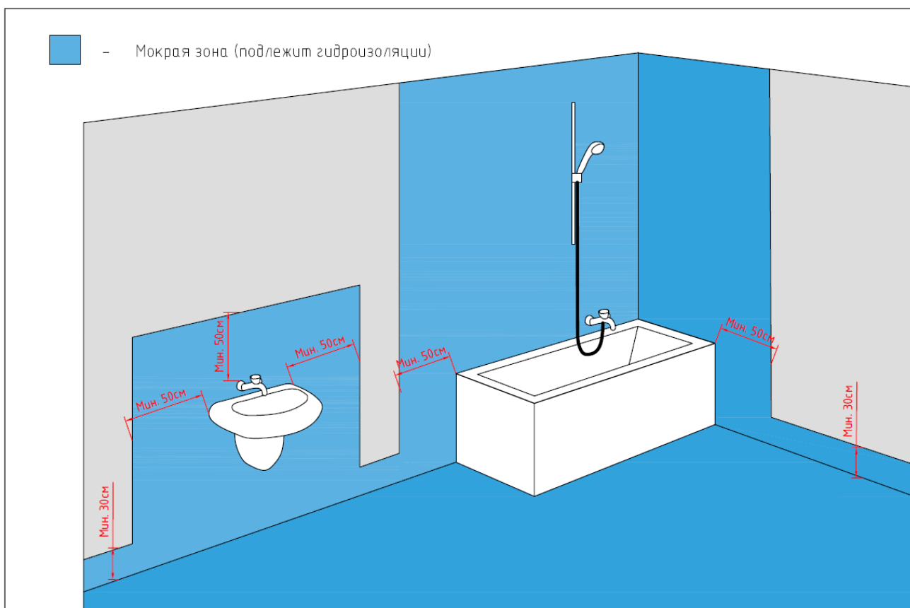
Рис. 32.2 Мокрые зоны внутри влажных помещений, подлежащие гидроизоляции.
