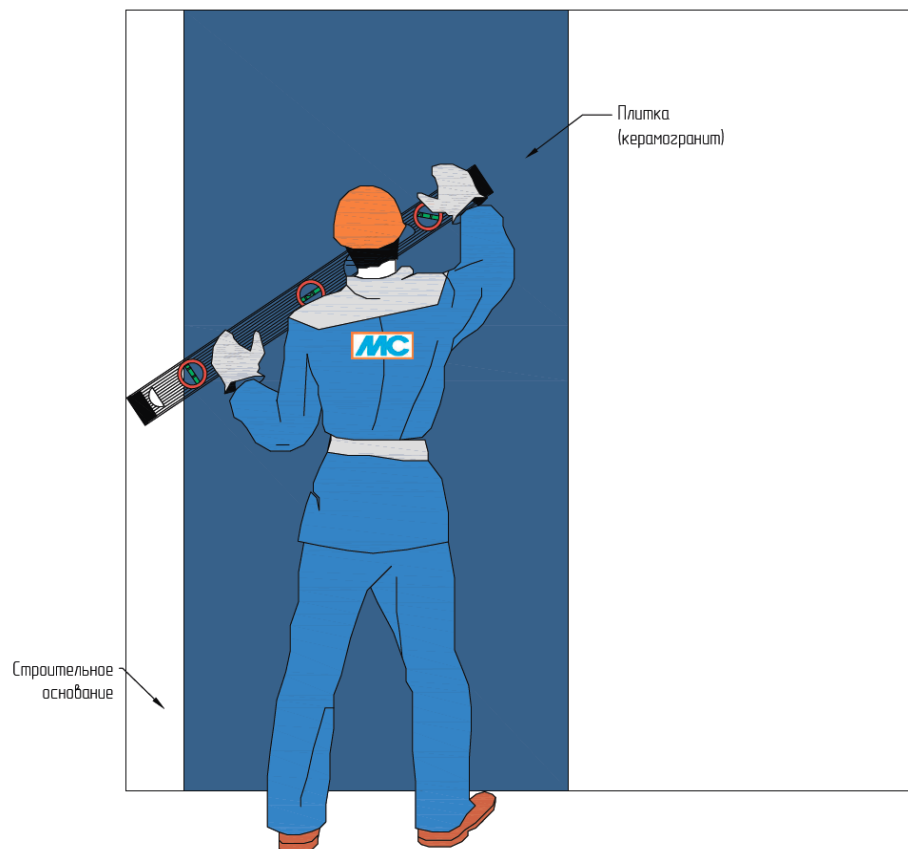
Рис. 40. Проверка облицовки при помощи уровня
